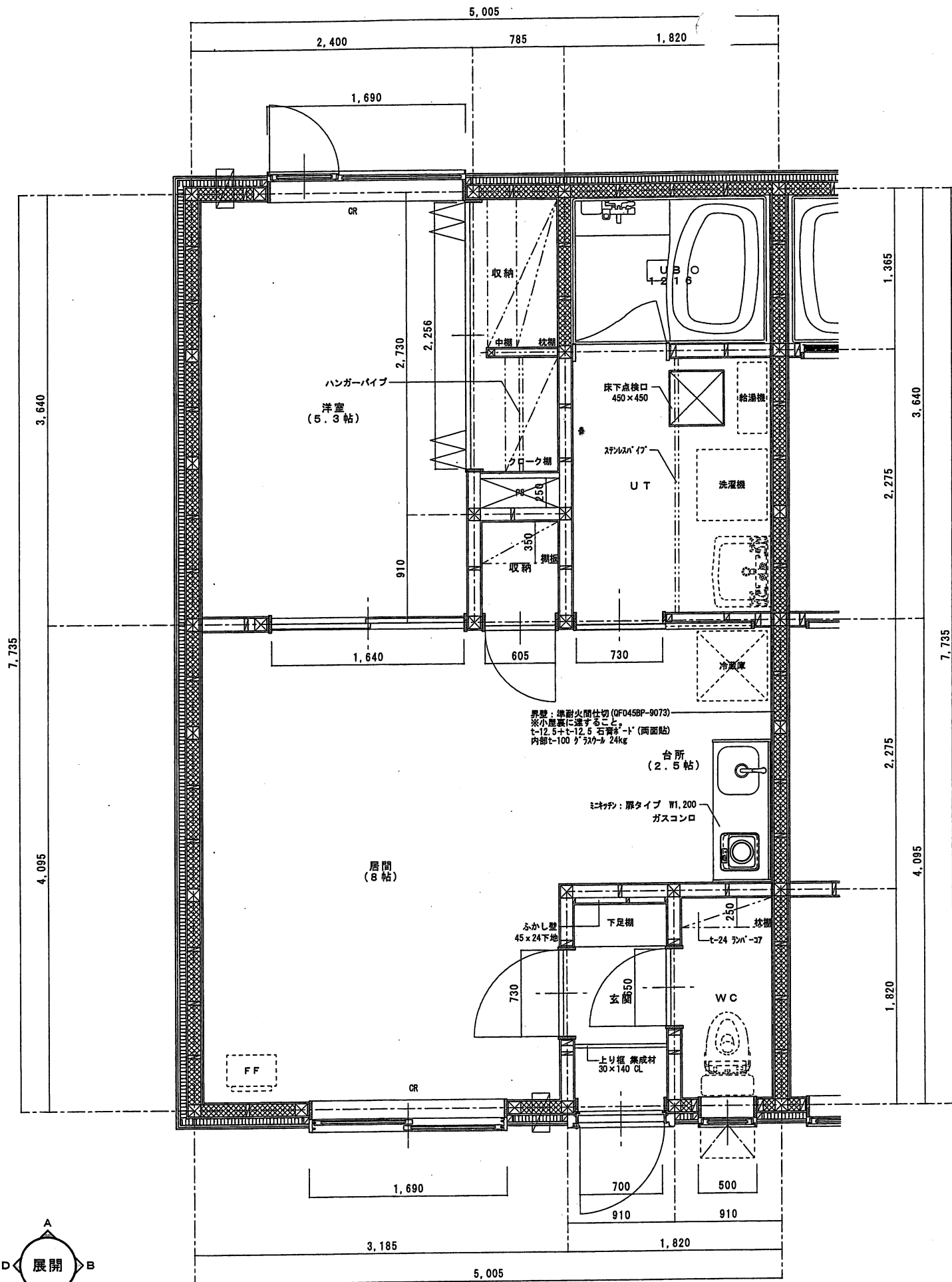
1F住戸平面詳細図
