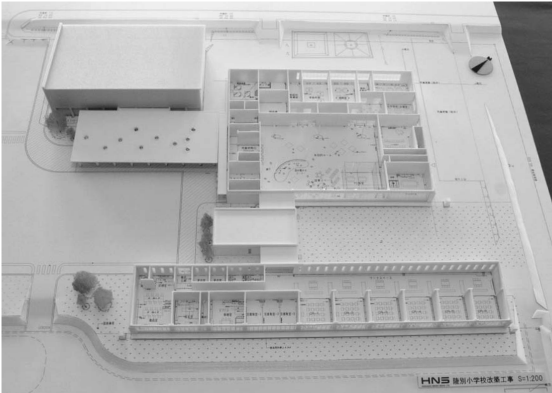
上は1/200の模型、左ページは平面図。
